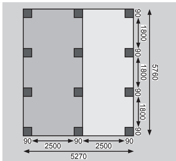
Carport + Abstellraum 3
