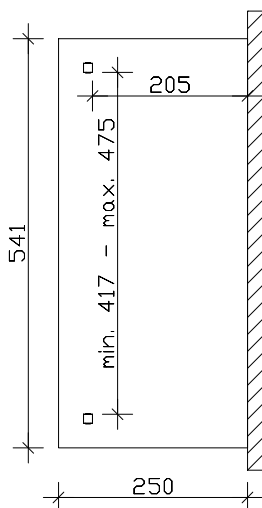
Grundriss
