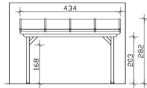
Frontansicht
