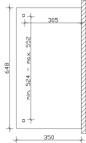
Grundriss
