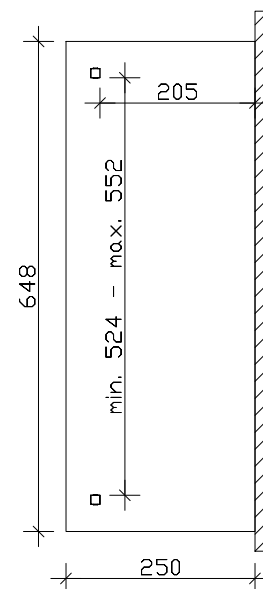
Grundriss
