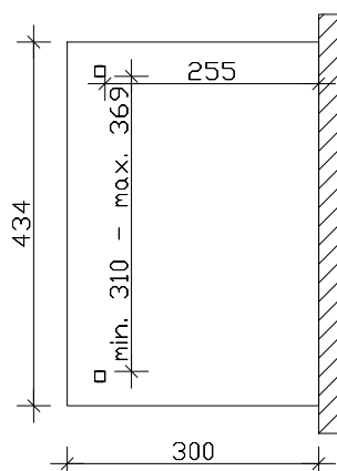
Grundriss
