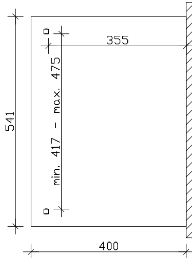
Grundriss
