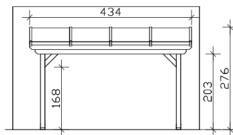
Frontansicht
