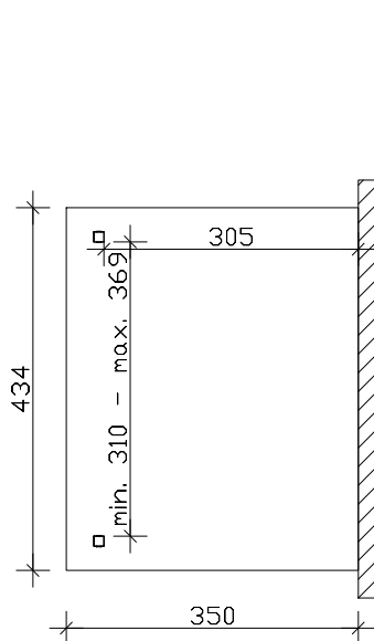
Grundriss
