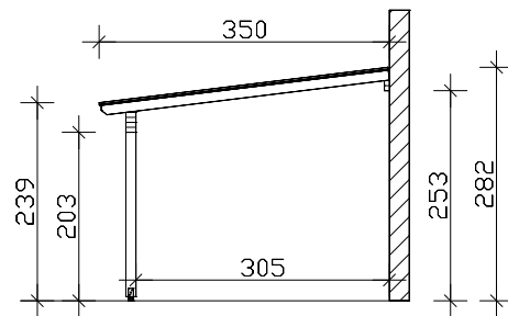
Seitenansicht
