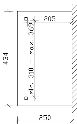
Grundriss
