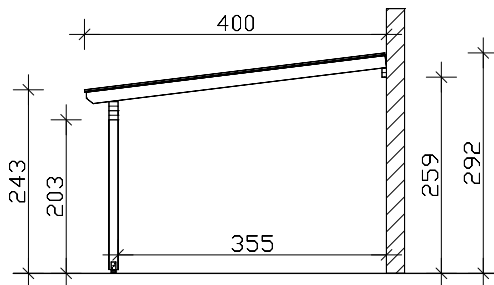
Seitenansicht
