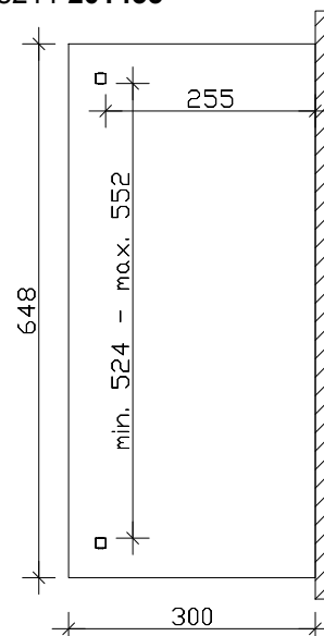
Grundriss
