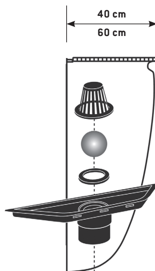
Montage der Geruchssperre MEASTOP für Lichtschächte Breite 40 oder 60 cm
