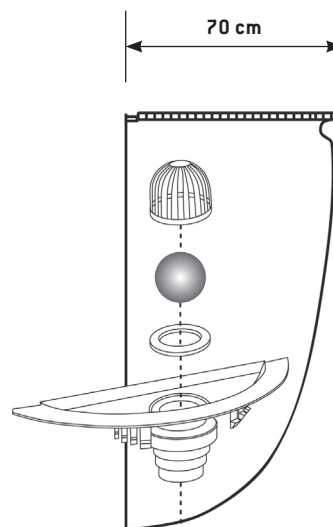
Montage der Geruchssperre MEASTOP für Lichtschächte Breite 70 cm
