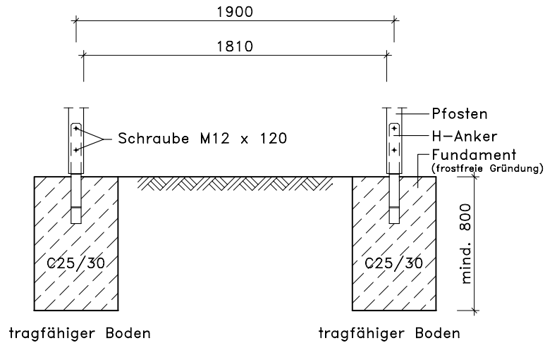
Schnitt A-A
