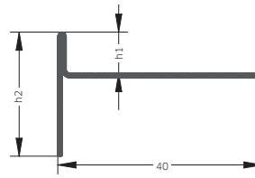
Beispiel: Ausführung rechts
