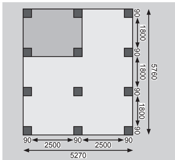
Carport + Abstellraum 1
