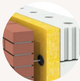
Ausführung mit Wärmedämmung & Luftschicht
