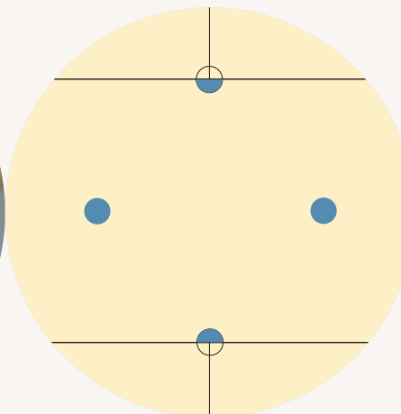
Dübelanordnung vier Stück pro Platte
