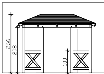
Frontansichten
