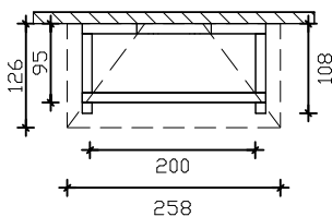
Grundrisse
