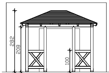
Frontansichten
