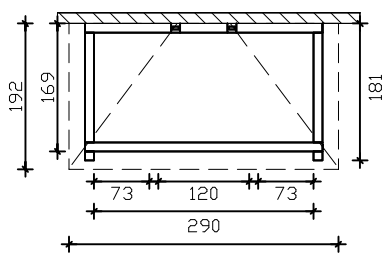
Grundrisse
