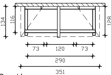
Grundrisse
