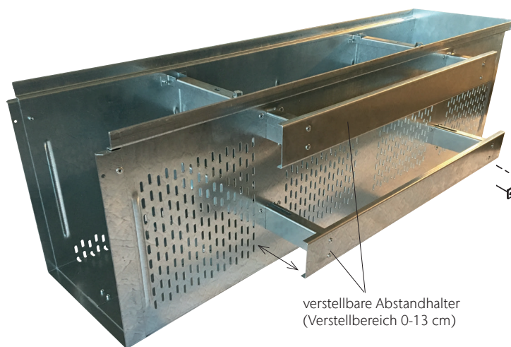
Ventilation durch Langlochraster
