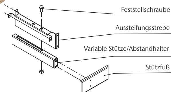
verstellbare Abstandhalter (Verstellbereich 0-13 cm)
