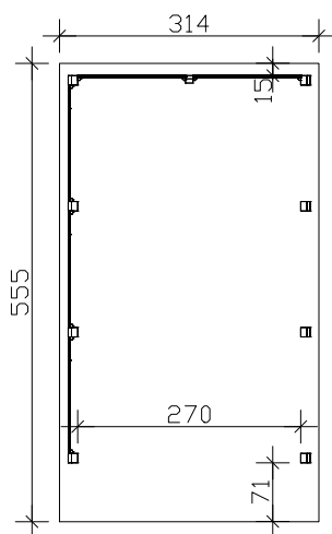
Grundriss
