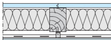
Skizze ohne Maßstab, ohne FTE, ohne unterseitige Beplankung
