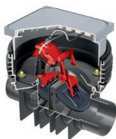
Rückstauautomat Quatrix
