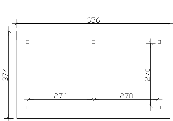
Grundriss (Gr.1)
