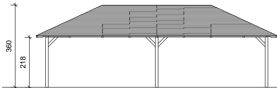
Frontansicht
