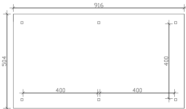
Grundriss (Gr.3)
