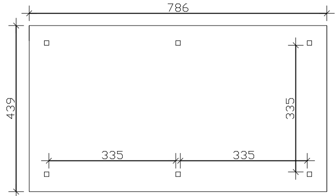
Grundriss (Gr.2)
