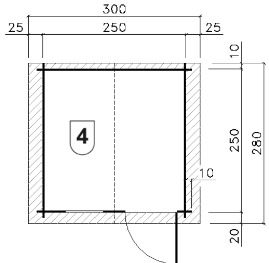
Angaben in cm
