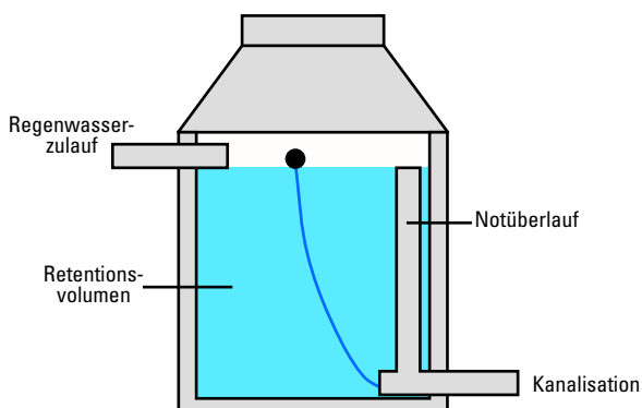
Aufbau eines Retentionstanks mit 100 % Regenwasser-Rückhaltung
