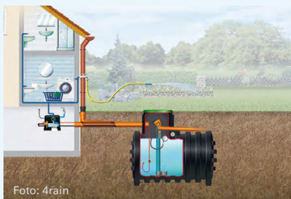
Foto: 4rain Regenwasseranlage zur Hauswassernutzung mit Anschluss an das Kanalnetz.
