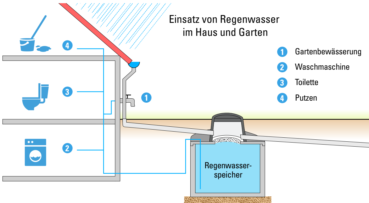
Einsatz von Regenwasser im Haus und Garten.
