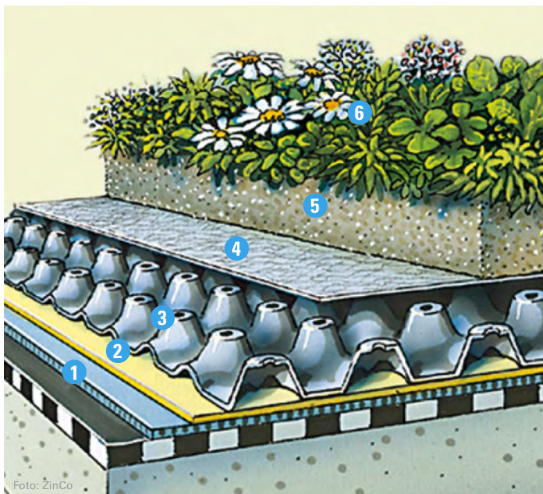
Aufbau Dachbegrünung
