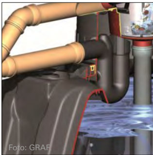
Foto: GRAF Überlaufsiphon
