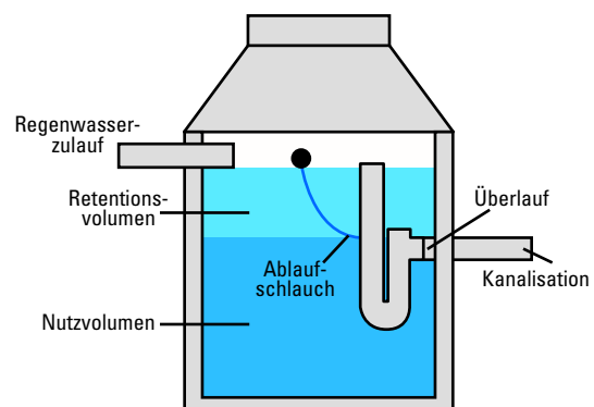
Aufbau eines Retentionstanks mit Regenwassernutzung kombiniert
